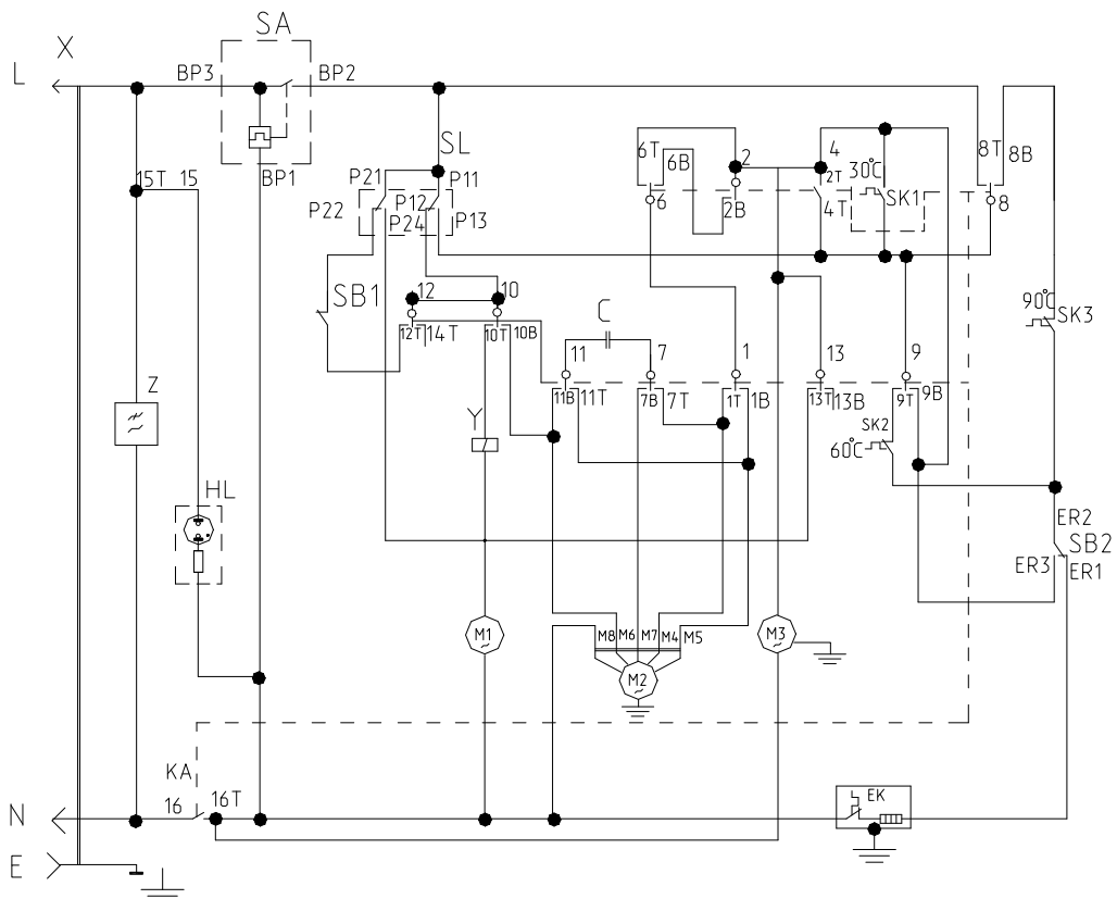
Рисунок В.1 - Схема электрическая принципиальная машины СМА-5ФБ 520-XX
