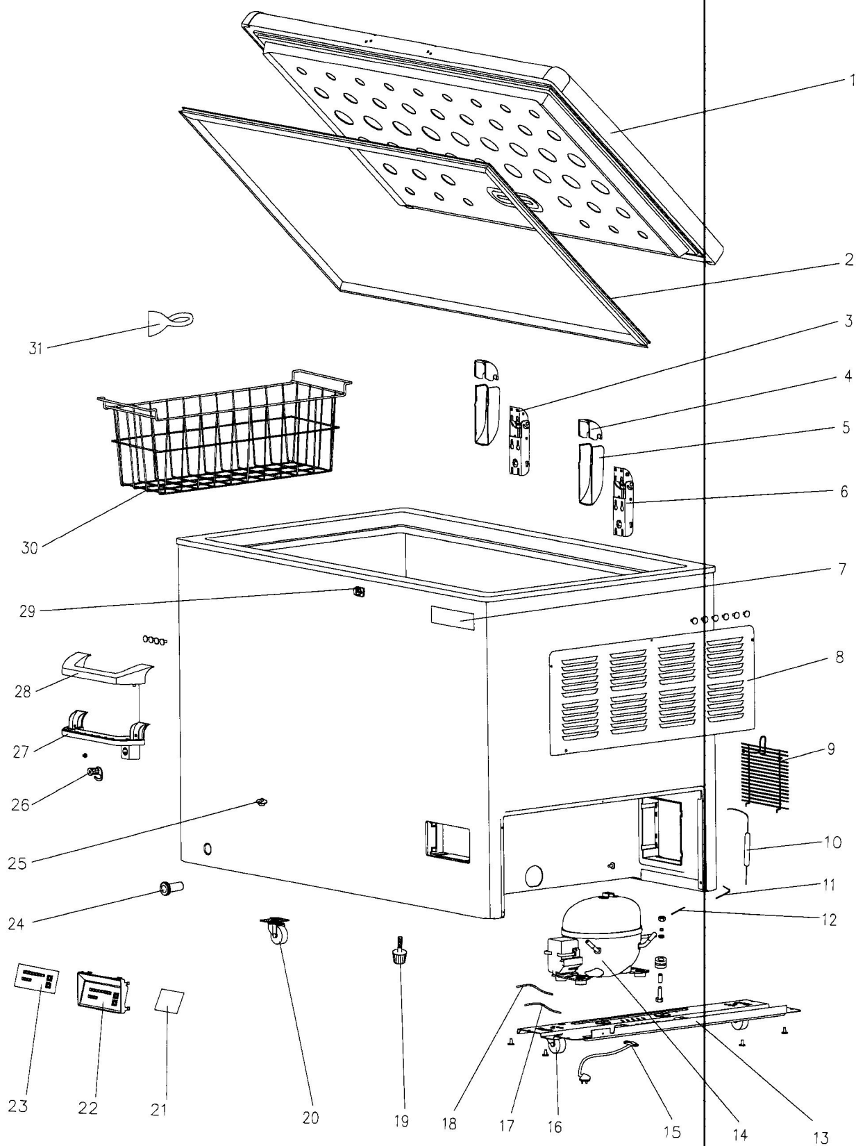
Рисунок 1 - Иллюстрации и перечень сборочных единиц
